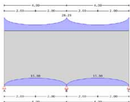
Bild 2. Eigengewicht und Anteil der unten angehängten Lasten
