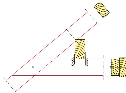
Bild 4. Kehlbalkenanschluss mit Pfette oberhalb
