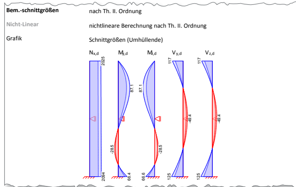
Bild 5. graf. Ausgabe der Bemessungsschnittgrößen
