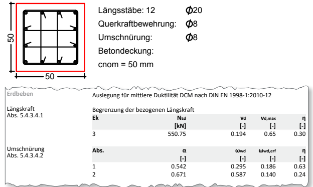
Bild 9. Erdbebennachweis in Duktilitätsklasse DCM
