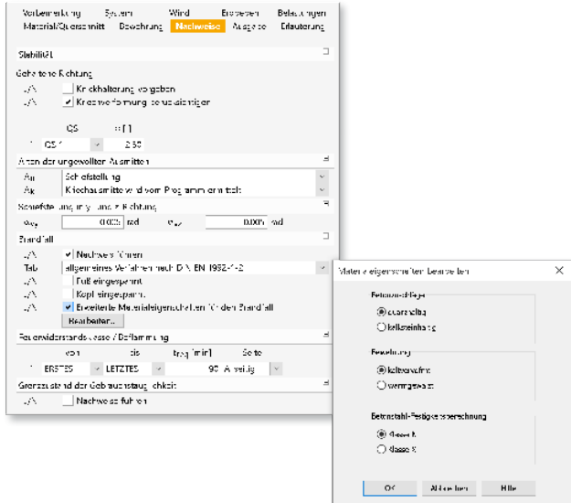
Bild 7. Erweiterte Eingabe Brandnachweise
