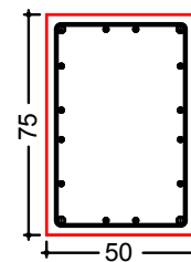
Bild 3. Beispiel für manuelle Bewehrungsanordnung
