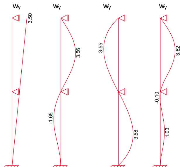
Bild 4. Beispiele für den Ansatz von Imperfektionen
