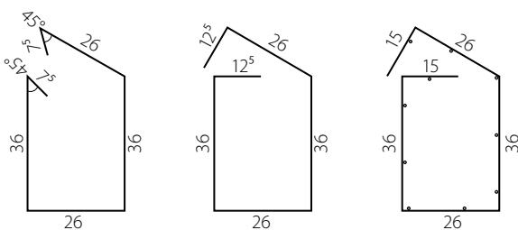
Bild 2. Biegeformen Rechteckbügel
