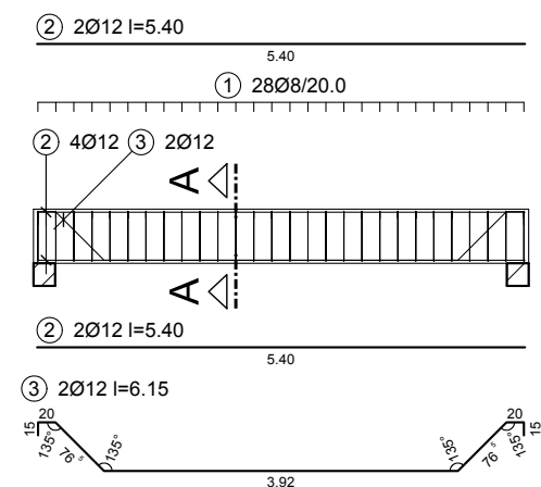
Bild 12. Feldbewehrung mit Schubaufbiegung
