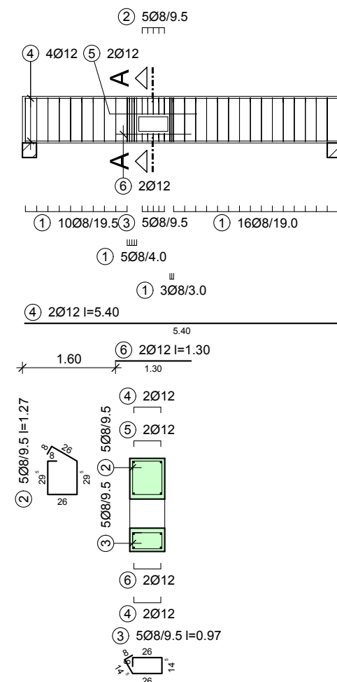
Bild 13. Bewehrungsdetails im Öffnungsbereich
