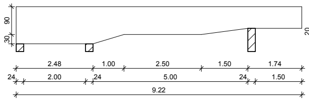
Bild 14. Schalplanausschnitt mehrfach gevouteter Träger
