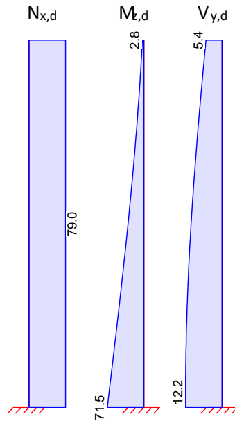
Schnittgrößen (je Kombination)
