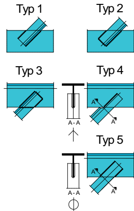
Bild 2. Verschiedene Anschlussausbildungen mit offenen Profilen ohne Knotenbleche
