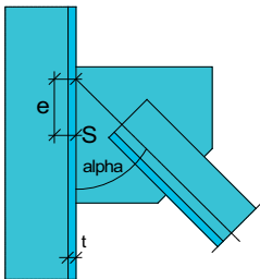
Bild 3a. Definition Anschlusswinkel
