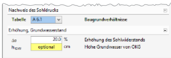
Bild 3. Auswahl der Tabelle für nichtbindigen Boden nach DIN 1054 zum Nachweis des ausreichenden Sohlwiderstandes und Eingabe einer prozentualen Erhöhung
