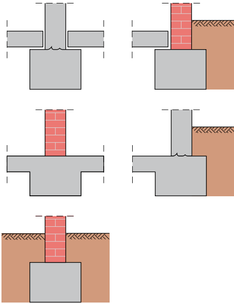
Bild 1. Mögliche Geometrie von zu berechnenden Streifenfundamenten
