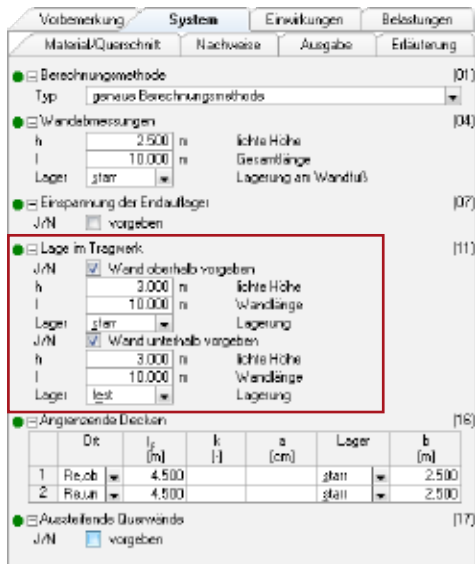
Bild 8. Systemeingabe mit Wänden ober- und unterhalb der betrachteten Wand
