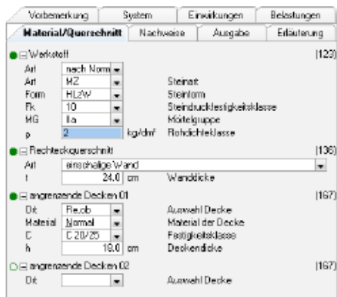
Bild 3. Materialdefinition von genormten Mauersteinen
