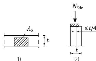
Bild 15. Maße und Bezeichnungen im Bereich von Teilflächenbelastungen
