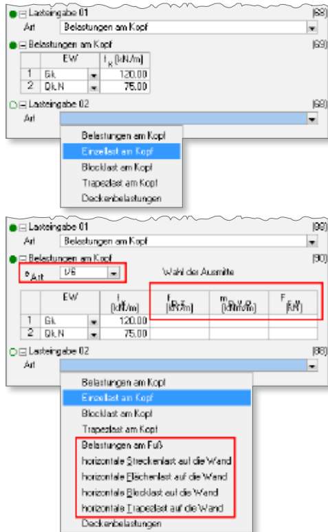
Bild 2. Angepasste Belastungseingabe, hier Unterschiede in der Lastdefinition
