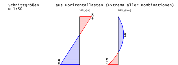
Bild 11. Schnittgrößen aus horizontaler Plattenbelastung
