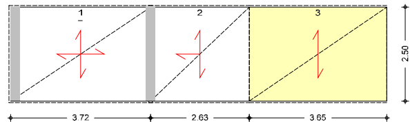
Bild 6. Automatische Aufteilung der Wand in Knicklängenbereiche
