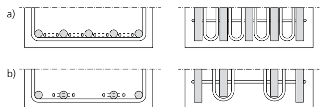
Bild 9. Anordnung Schlaufen a) zwischen vorhandener Bewehrung b) einem vorhandenen Bewehrungsstabe zugeordnet
