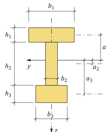
Bild 4. Bezeichnungen für einen Doppel-T-Querschnitt
