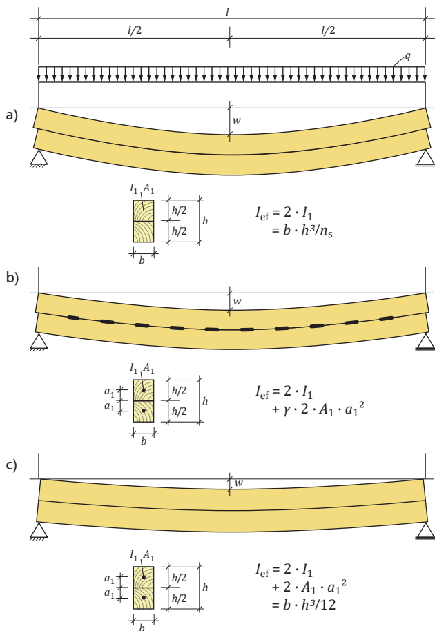
Bild 1. Tragverhalten eines Biegeträgers aus zwei Holzquerschnitten a) kein Verbund b) nachgiebiger Verbund c) voller Verbund
