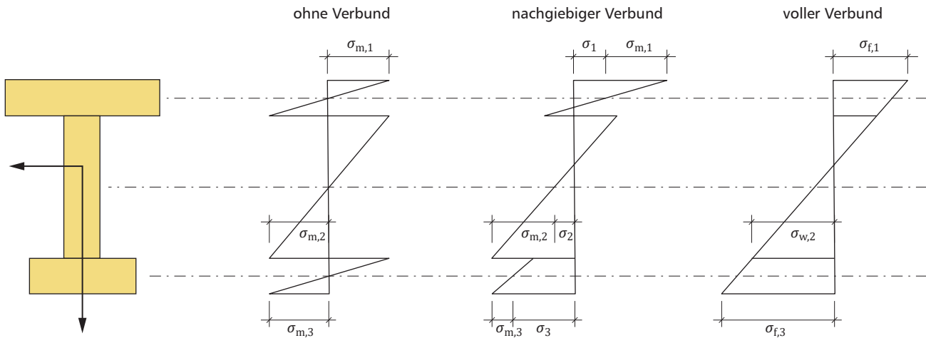
Bild 3. Prinzipieller Spannungsverlauf für einen Doppel-T-Querschnitt mit unterschiedlichem Verbund
