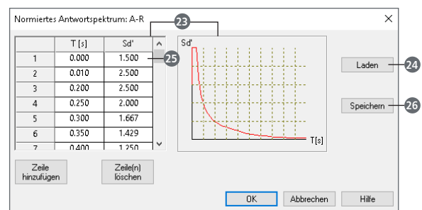
Bild 10. Bemessungs-Antwortspektrum
