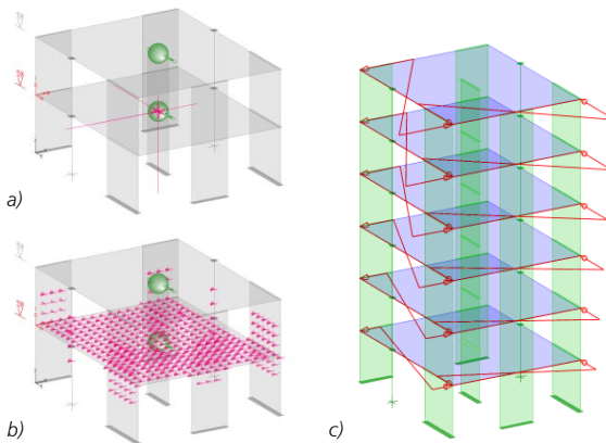
a) Ersatzlasten im selektierten Auswertungsraum b) Konzentrierte Lasten im Lastzentrum c) Zusätzliche Lasten zur nicht planmäßigen Torsionswirkung
