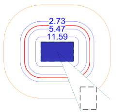
Erforderliche Durchstanzbewehrung je Rundschnitt an Rechteckstütze
