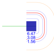
Erforderliche Durchstanzbewehrung je Rundschnitt an Wandende
