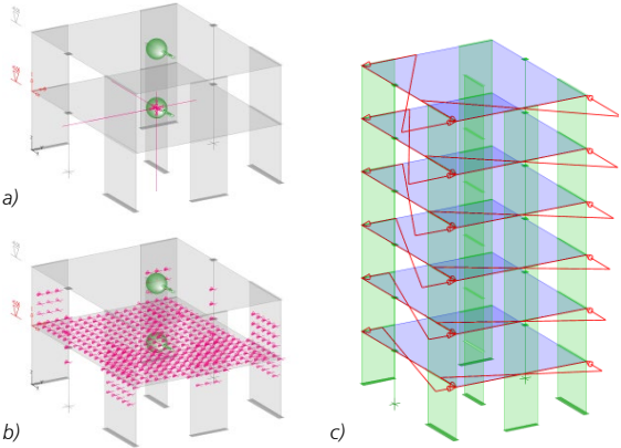
a) Ersatzlasten im selektierten Auswertungsraum b) Konzentrierte Lasten im Lastzentrum c) Zusätzliche Lasten zur nicht planmäßigen Torsionswirkung
