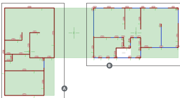
Bild 5. Deckensystem über zwei Gebäudeteile
