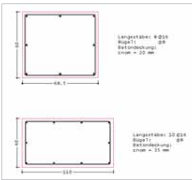
Bild 6. Grafische Darstellung der gewählten Längsbewehrung
