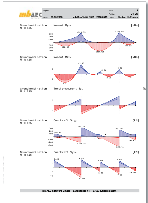
Bild 4. Ausgabe der Bemessungsschnittgrößenverläufe
