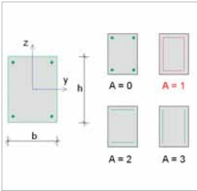
Bild 5. Grafische Hilfe „Bewehrungsanordnung“
