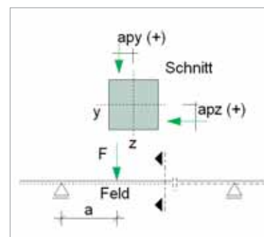
Bild 3. Grafische Hilfe „ausmittiger Lastangriff“
