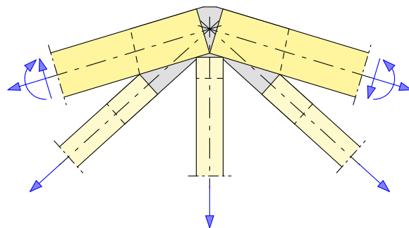
Bild 2. Schematische Darstellung der Belastung auf das System
