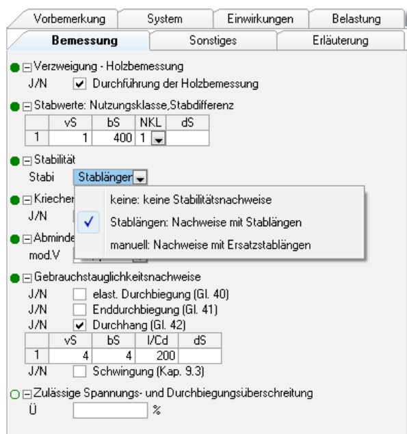
Bild 3: Eingaberegister „Bemessung“
