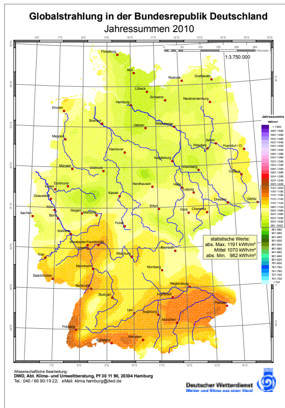
Bild 6. Jahressummenverteilung der kWh/m 2 und möglicher Maximalertrag nach Ausrichtung und Dachneigung ( www.dwd.de/globalstrahlung )
