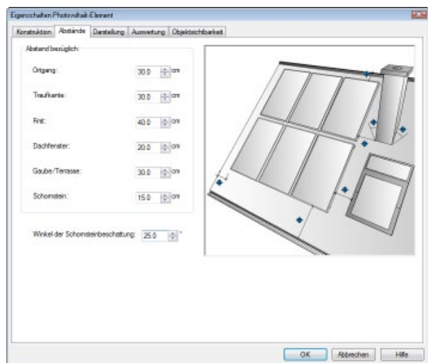
Bild 4. Konstruktions- und Verlegedaten als Bauteileigenschaften
