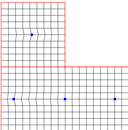
Bild 7. Vernetzung
