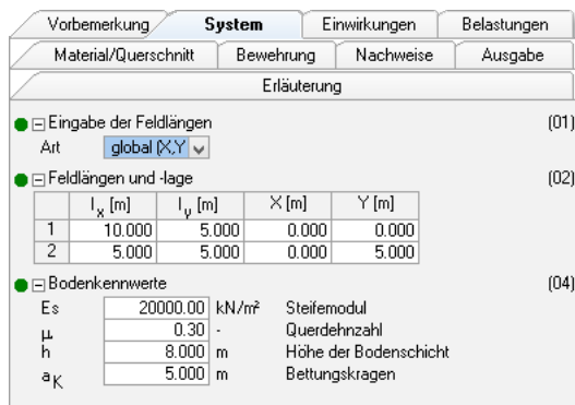
Bild 2. Kapitel „System“
