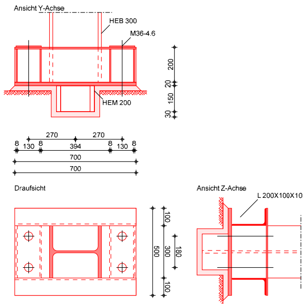
Bild 4. Fußausbildung mit Traverse und durchgehender Fußplatte
