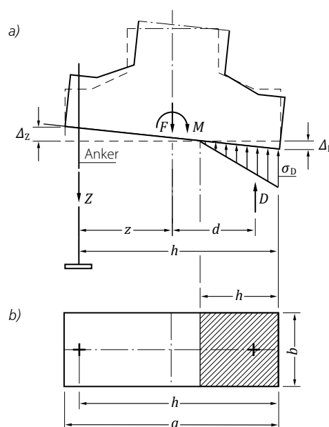
Bild 2. Berechnungsansatz nach Petersen, Bild 90, [9]
