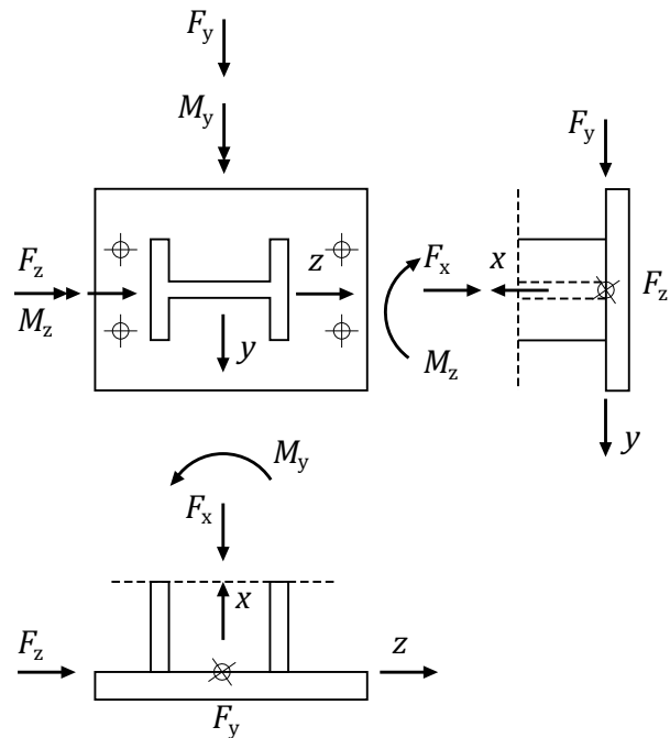
Bild 3. Graf. Hilfe, Eingabe der Auflagerlasten
