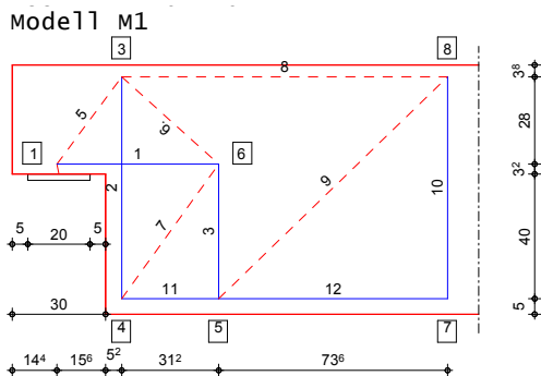
Bild 1. Fachwerkmodell M1
