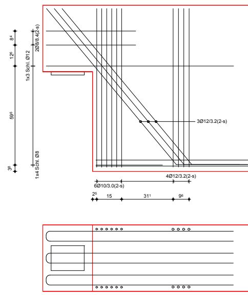
Bild 8. Bewehrungsgrafik
