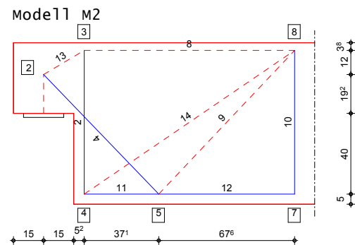
Bild 2. Fachwerkmodell M2
