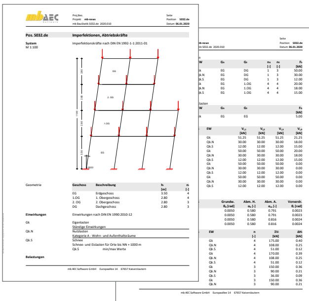
Bild 4. Beispielausgabe von Imperfektionskräften
